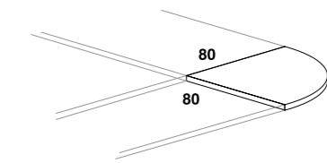
UNIÓN ANGULAR 90° 80 / 80. 90°CONNECTOR 80/80. ANGLE LIAISON 90° 80 / 80.
